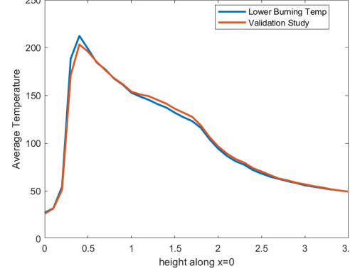
(d) Recorded temperature at x=0
