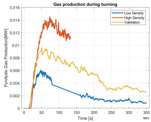
(d) Pyrolysis gas formation Density
